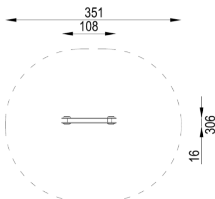
Widok urządzenia
