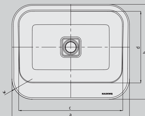
Wariant zabudowy A* (szerszy rant = przednia strona umywalki)
