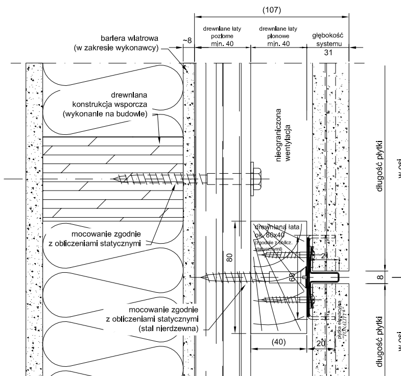
przekrój poziomy
