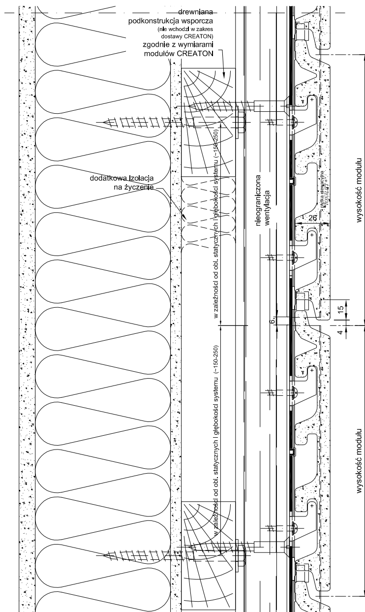
przekrój pionowy
