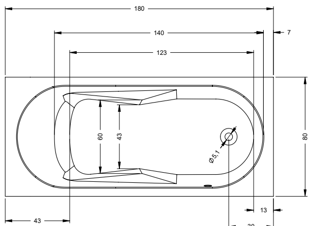
WANNA LAZY PRAWA (przelew po prawej stronie) BC42 180x80 cm
