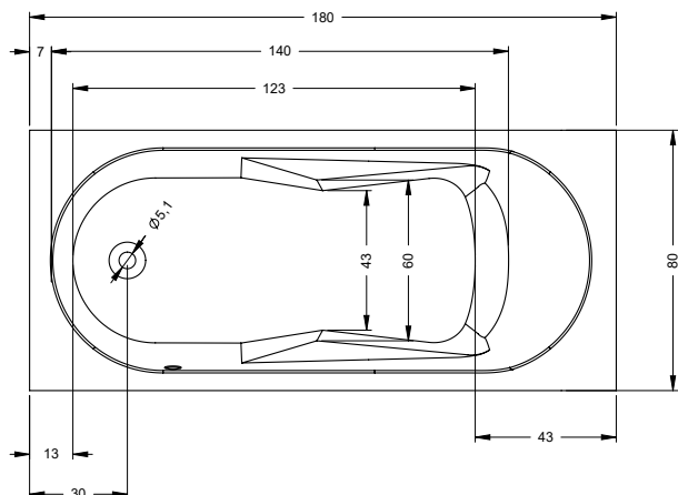
WANNA LAZY LEWA (przelew po lewej stronie) BC43 180x80 cm
