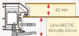
Schemat zespoleńia ościeżnicy ze skrzydłem 3D
