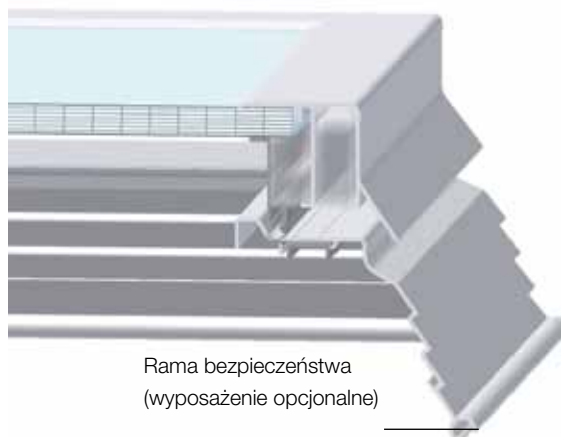
Przekrój Kingspan Classic PC-s Dome
