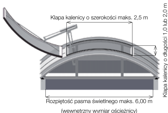
Pasma świetlne basic Kingspan ESSMANN w przekroju
