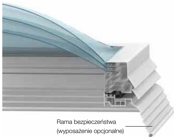
Światlik kopułkowy classic 3-warstwowym w przekroju
