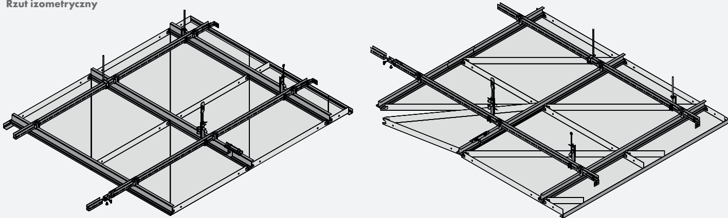
Rzut izometryczny
