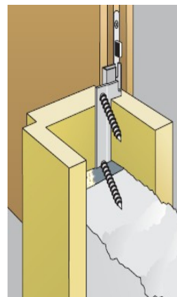
Przykład montażu ościeżnicy F97m na dyble z zaprawą betonową.
